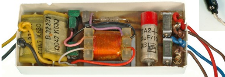
Miniature AC mains unit 33217-20.
